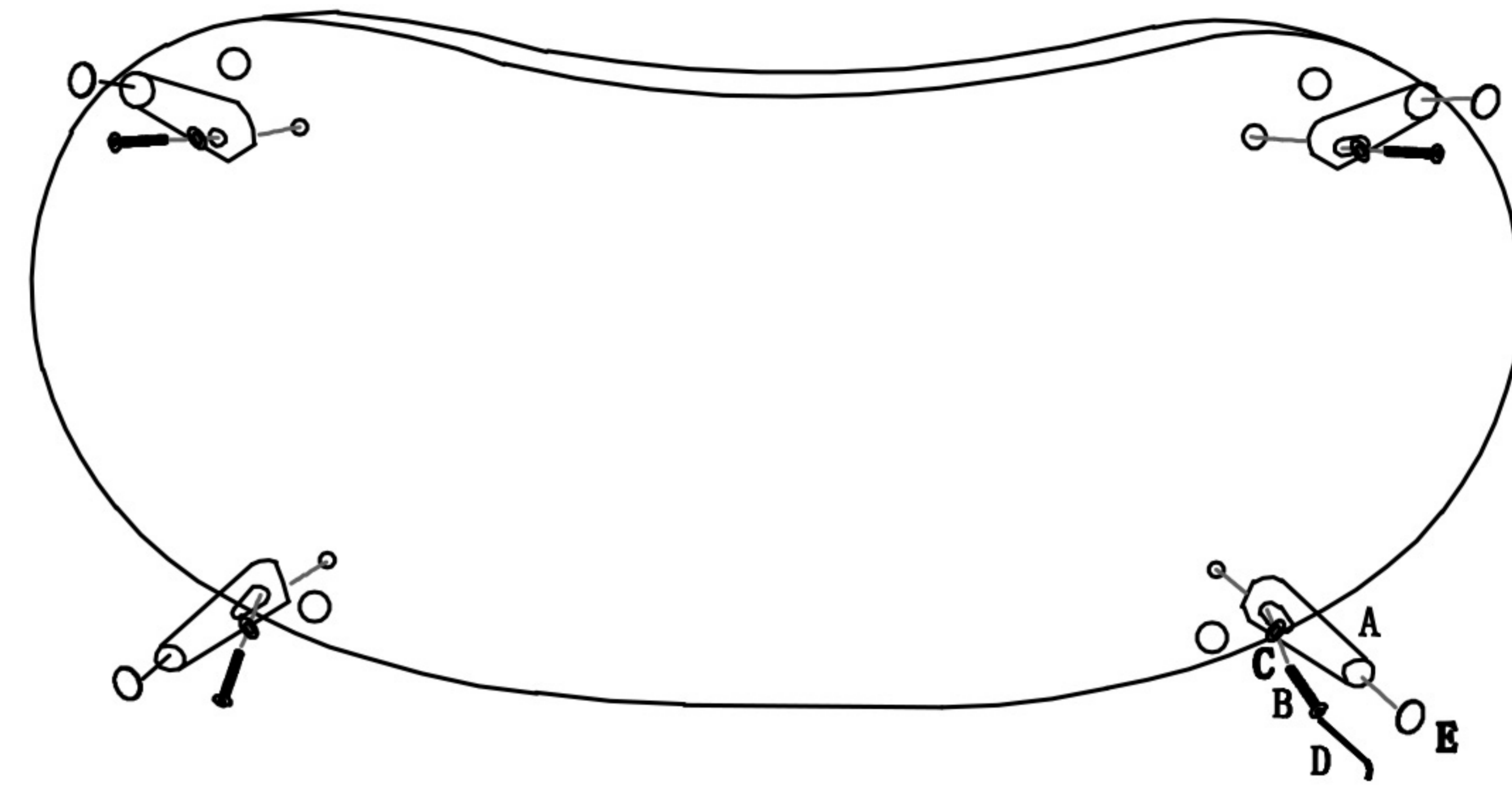
脚取付図
